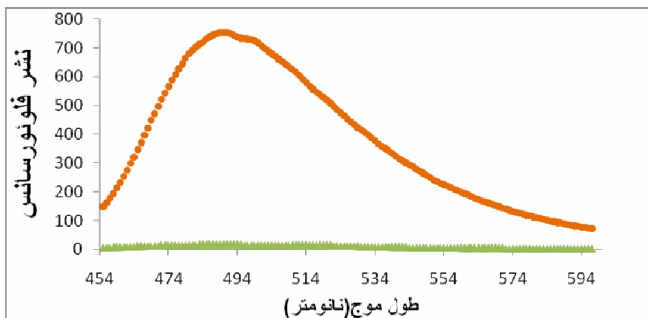
شکل ۲- طیف جذبی کنگورد (□)، پس از اضافه کردن آلبومین سرم انسانی انکوبه شده به مدت ۲۴ ساعت در pH=۱/۵ و دمای ۵۷ درجه سانتی گراد (+) و در مجاورت آلبومین سرم انسانی انکوبه نشده (□).
