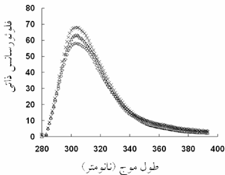
شکل ۲- طیف نشری فلورسانس ذاتی انسولین طبیعی (×) و سیتراکونیل شده (◊) و سیتراکونیک آنهیدراید ۱ میلی مولار، Δ: سیتراکونیک آنهیدراید ۲ میلی مولار در pH=۷/۵. طول موج برانگیختگی ۲۸۰ نانومتر بود.
