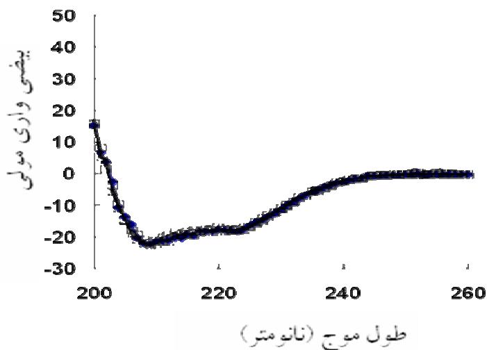
شکل ۳- طیف جذبی دورنگ نمایی دور انسولین در pH=۷/۵ نمونه طبیعی (◊) و تغییر داده شده با سیتراکونیک آنهیدراید ۱ میلی مولار (□) و ۲ میلی مولار (Δ). (واحد بیضی واری مولی \text{degree. cm}^2. \text{dmol}^{-1} است).
