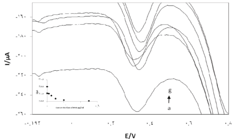
شکل ۷- ولتاموگرام‌های تمایز پالسی برای تشخیص HSA بر اساس رقت‌های سریالی مختلف آنتی‌ژن (a تا g) (۰/۰۵، ۰/۲، ۰/۵، ۱، ۲، ۵، ۱۰، ۲۰، ۵۰، ۱۰۰، ۲۰۰، ۵۰۰، ۱۰۰۰ µg/ml) در HCl یک مولار در سرعت خوانش ۵۰ mV/s
