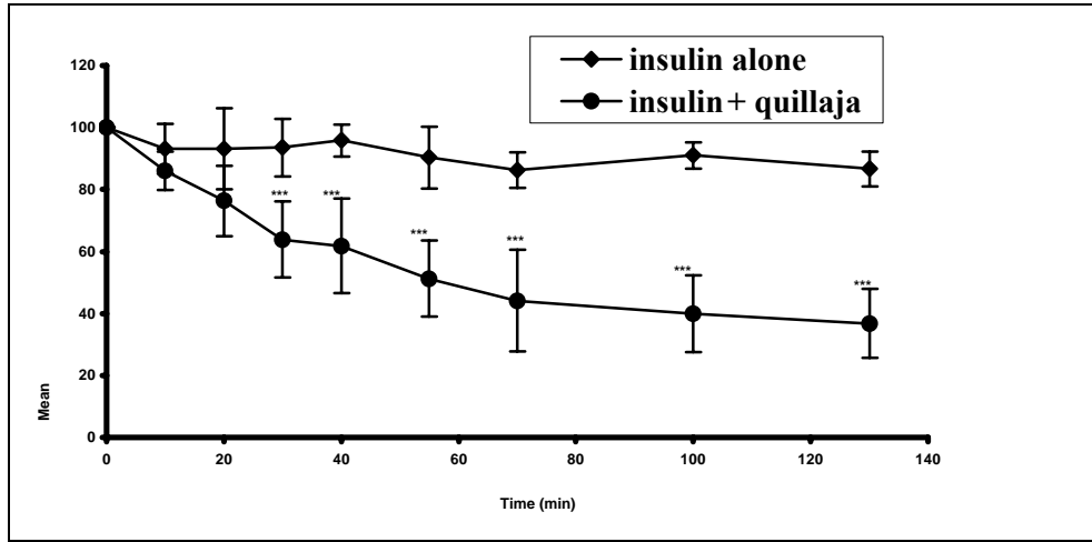
شکل ۲ - میانگین غلظت گلوکز خون نسبت به زمان پس از تجویز داخل بینی محلول حاوی ۲ واحد انسولین رگولار (♦) و محلول حاوی ۲ واحد انسولین رگولار به همراه ۱٪ ساپونین تام کیلیا (●) در رت (n=۵). نتایج به صورت انحراف معیار ± میانگین گزارش شده‌اند.
