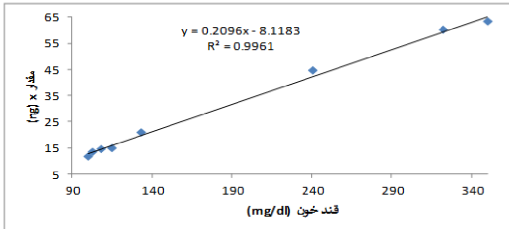
شکل ۷- نمودار همبستگی میزان استون بازدم تنفسی (داده‌های حاصل از روش طیف‌سنجی تحرک یونی) و قند خون بیماران دیابتی
