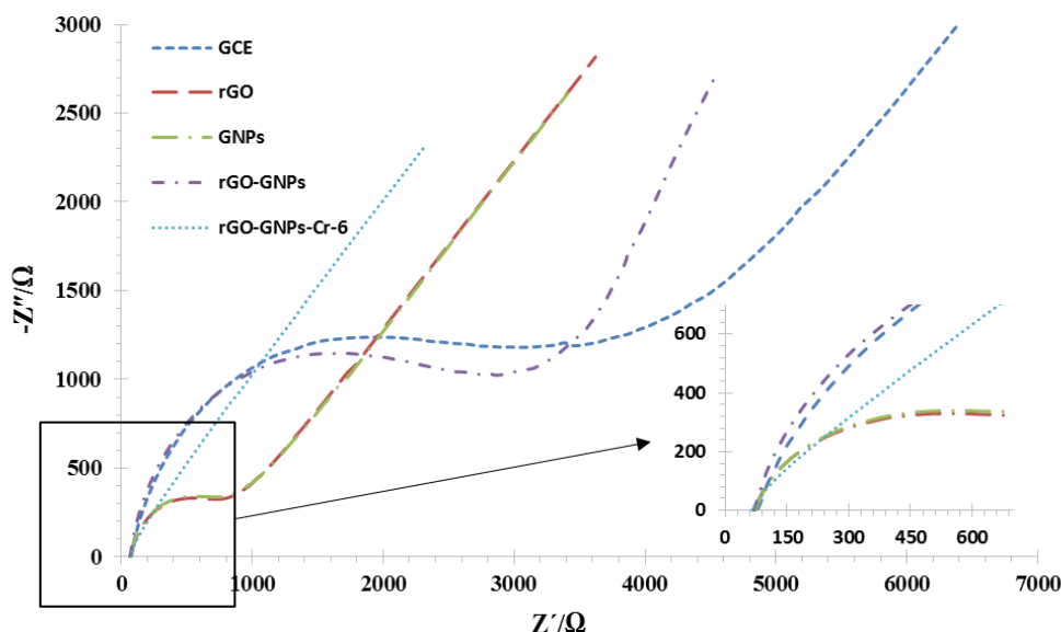
شکل ۴- نمودار نایکوئیست ثبت شده در پروب کلرید پتاسیم ۵ میلی مولار و همچنین فروسیانید آهن \text{Fe}(\text{CN})_6^{4-} ۲۵۰ میلی مولار با استفاده از GCE، rGO/GCE، rGO-GNPs/GCE و rGO-GNPs-Cr.6/GCE (دامنه فرکانس از ۱ هرتز تا ۱۰۰ کیلوهرتز)
