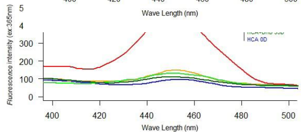
شکل ۳- طیف نشر فلئورسانس AGEs
