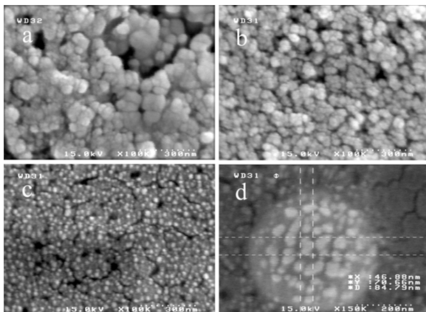
شکل ۲- تصاویر SEM از ایمونوسنسور (a) PVA (b) PVA-HSA (c) الکتروکود تغییر یافته PVA-HSA-AuNPs - (d) توزیع نانوذره طلا بعد از تشکیل Ab-AuNPs
