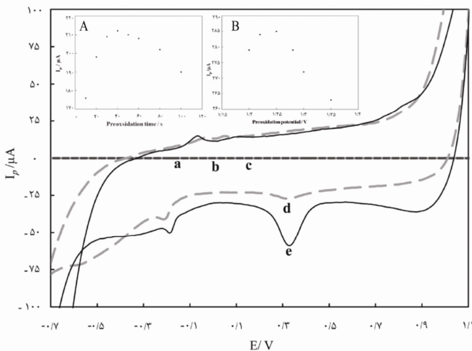
شکل ۳- انواع اشکال الکتروکود تغییر یافته در حضور HCl یک مولار در محدوده پتانسیل -۰/۷ تا +۱/۱ ولت. سرعت خوانش: ۵۰ mV/s (a) الکتروکود برهنه- (b) PVA (c) PVA-HSA (d) PVA-HSA-AuNP (e) PVA-HSA-AuNPs ولتاموگرام‌های تمایز پالسی پاسخ الکتروکود تغییر یافته برای بهینه سازی زمان الحاق: (a) (۱۰، ۲۰، ۳۰، ۴۰، ۵۰، ۶۰، ۷۰، ۸۰، ۹۰) ثانیه (b) پتانسیل (۱/۲۲/۲، ۱/۱، ۲۵/۱، ۱/۲۷، ۱/۳۰، ۱/۳۵، ۱/۴۰ ولت)
