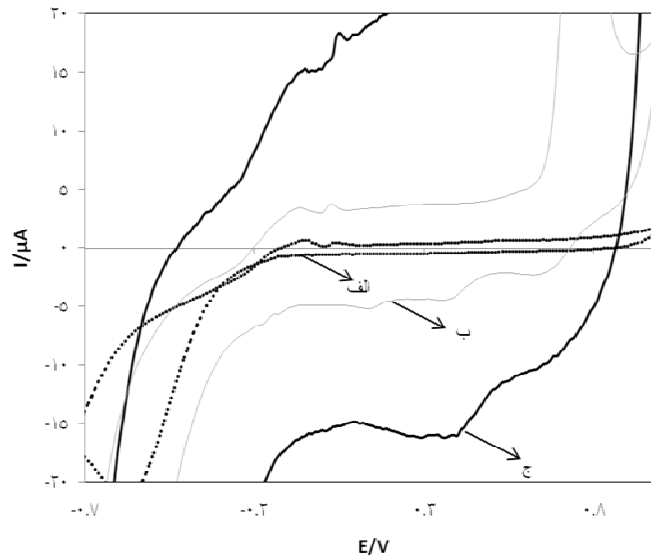
شکل ۵- انواع اشکال الکتروود تغییر یافته در حضور HCl یک مولار در محدوده پتانسیل -۱ تا +۱ ولت سرعت خوانش: 50 \text{ mV/s} . (a) الکتروود برهنه (b) PVA-HSA (c) PVA-HAS-Ab-MnG
