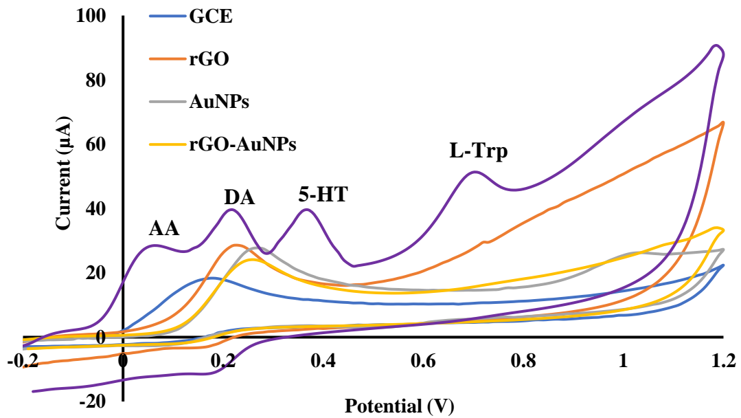
شکل ۷-سنجش سروتونین در حضور مواد مشابه جهت نمایش انتخاب‌پذیری سیستم با استفاده از الکترودها مختلف شامل GCE، rGO/GCE، AuNPs/GCE، rGO-GNPs/GCE و rGO-GNPs-Cr.6/GCE به روش CV
